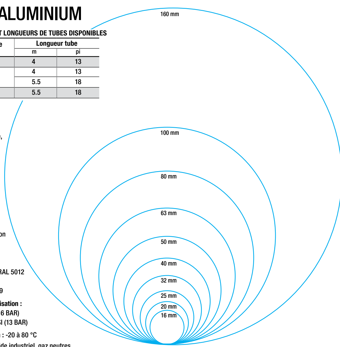
DIAMÈTRES RÉELS DES TUBES
