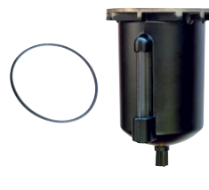
No de produit 50.850 Bol en métal + voyant (purreur auto) F 3/4 à 2 HIFLO
